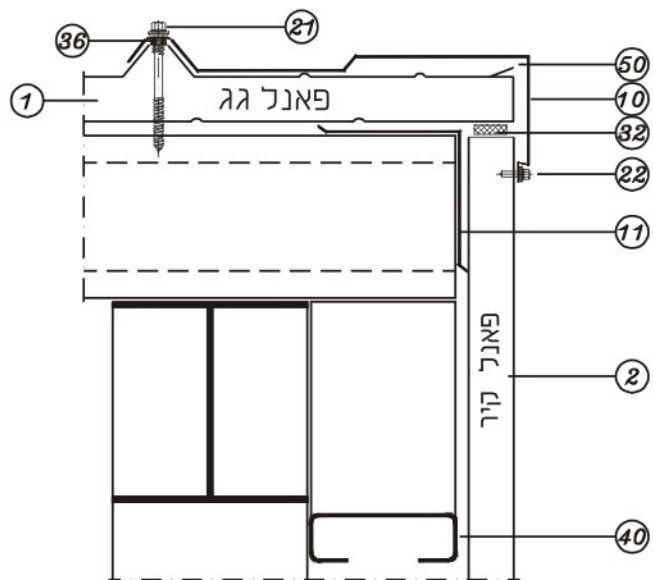
23A. חיבור גג לקיר גמלון
