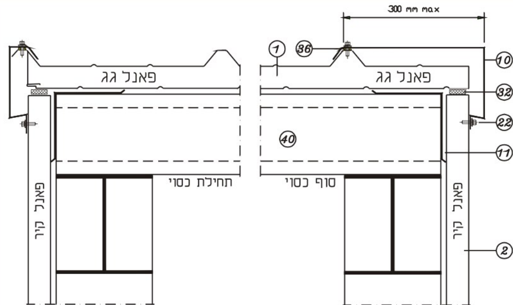
23A. חיבור גג לקיר גמלון
