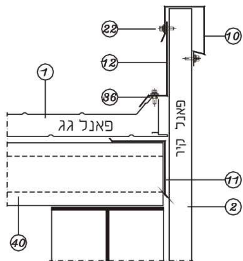
24א. חיבור גג לקיר גמלון מוגבה*
