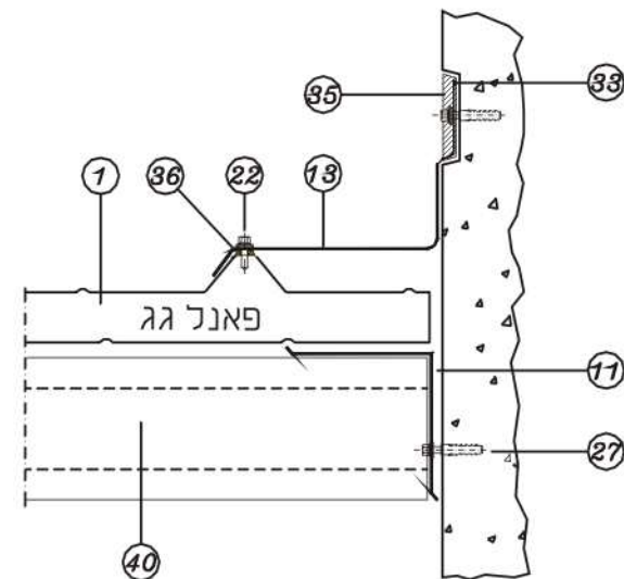
24B. חיבור בין גג לקיר קשיח*
